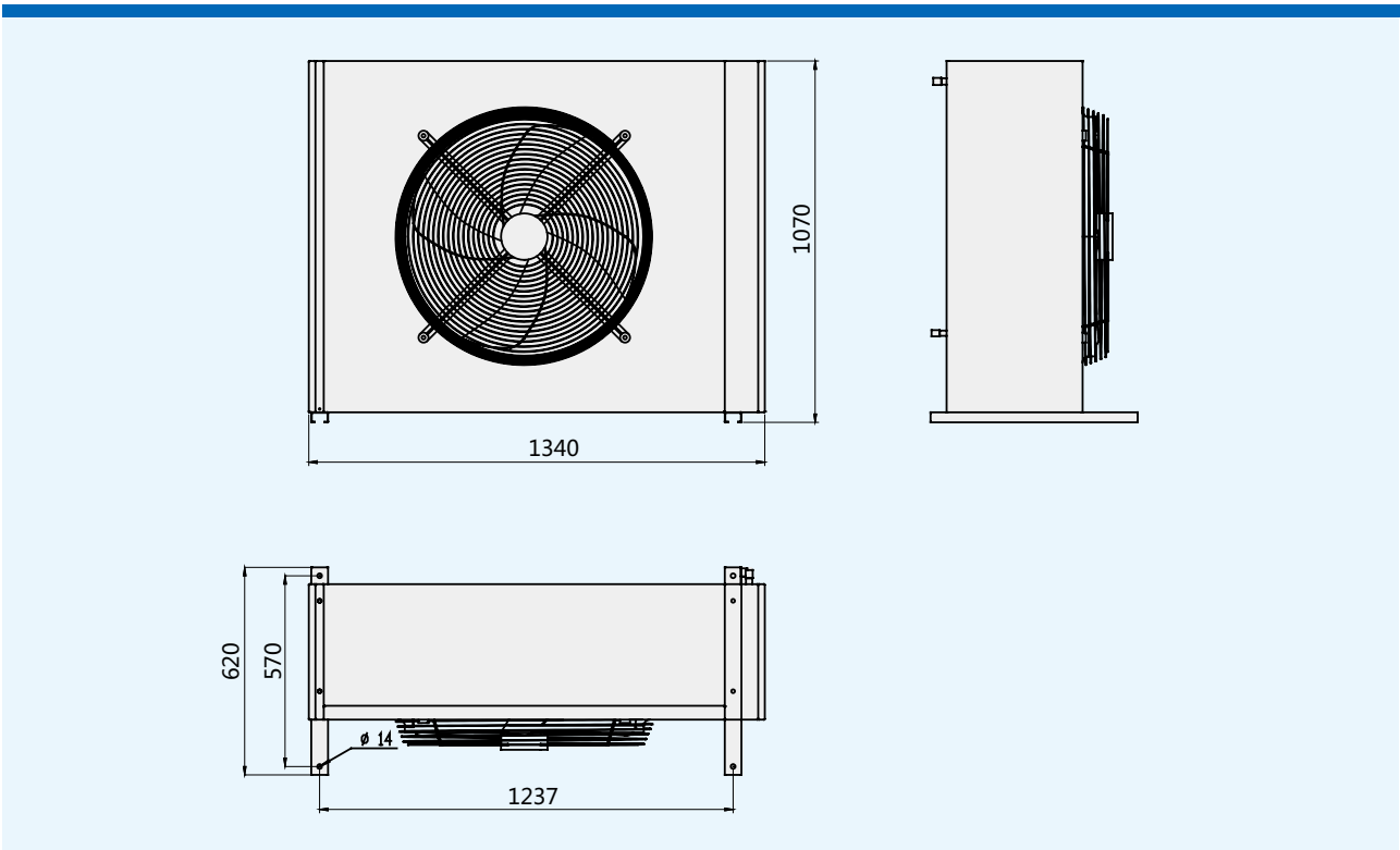
CMEG8/CMEG10 dimension drawing
